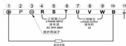
11KW主回路接线图:
