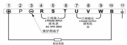
11KW主回路接线图:
