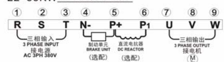
22-55KW主回路端子接线图:
