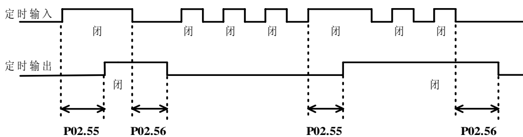
图 6.3.15 定时器功能图
