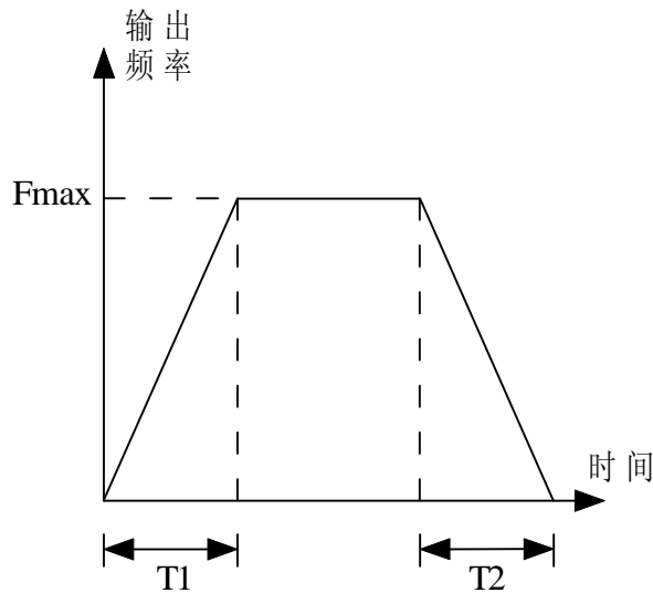
图6.1.9 加、减速时间的定义
