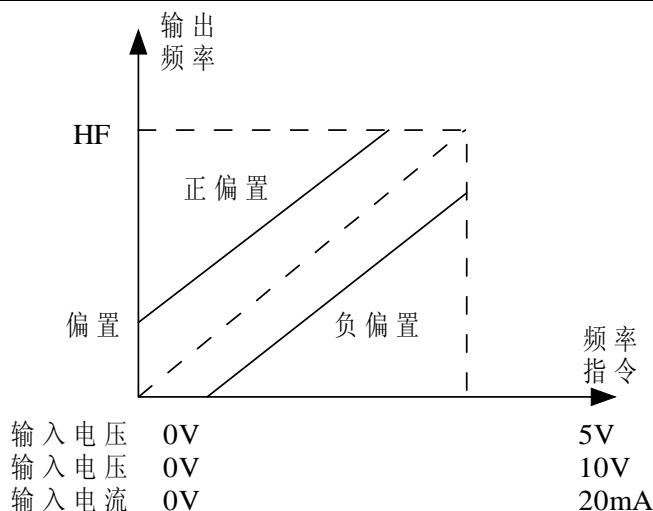
图6.2.4 偏置频率
