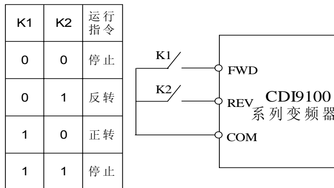
图6.3.6 两线控制模式 1
