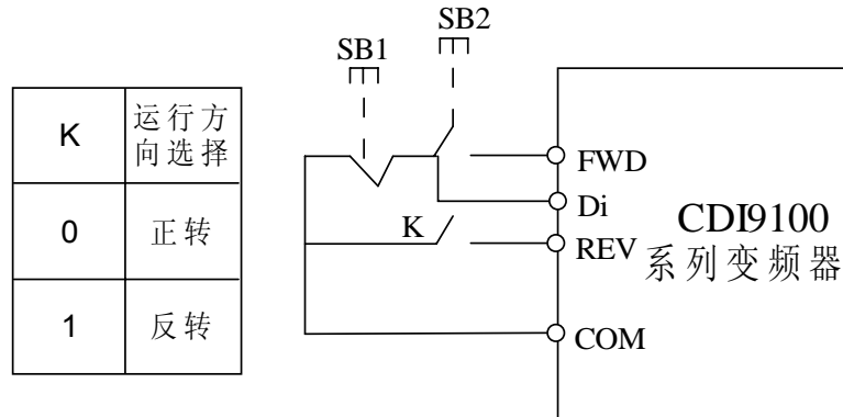
图 6.3.8 三线控制模式
