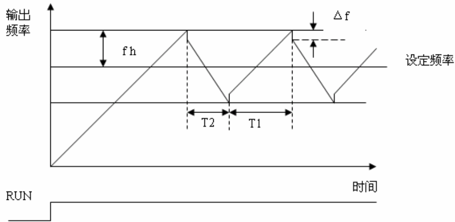
图 6.3.14 摆频运行图
