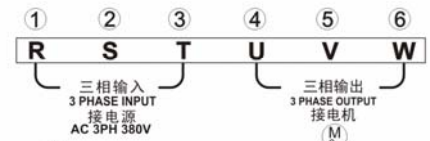
主回路接线图:
